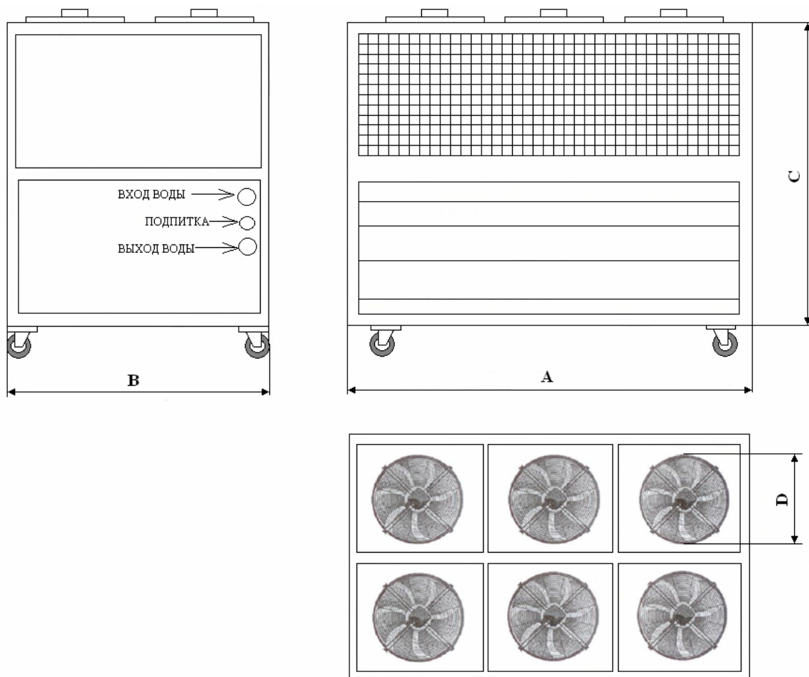
Рис.2. Габаритные размеры устройств
