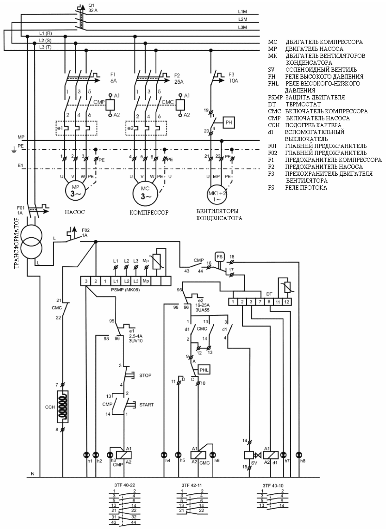
Рис.3. Принципиальная электрическая схема подключения охладителя
